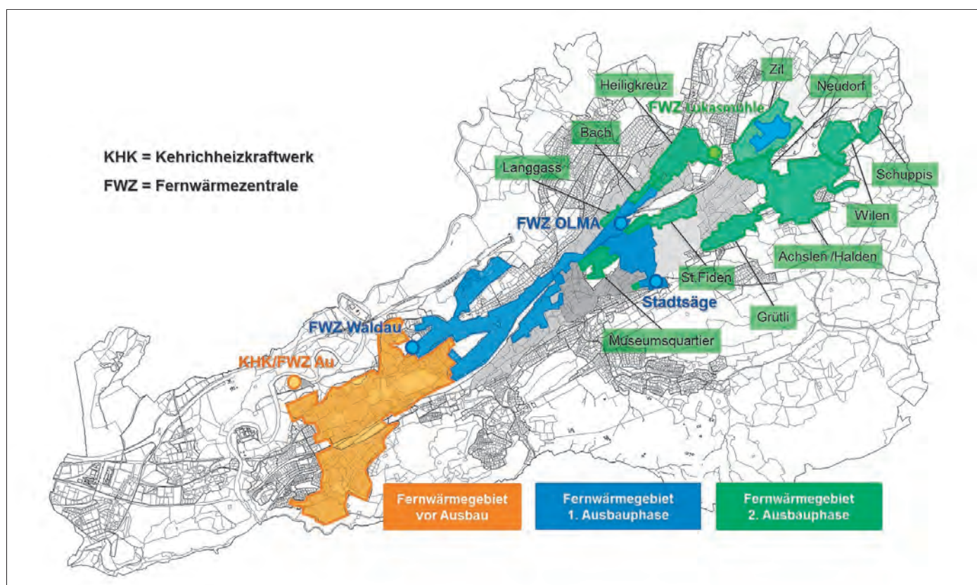
Abb. 1: Ausbau der städtischen Fernwärme St. Gallen. Die 2. Ausbauphase wurde im November 2017 vom Volk bewilligt.
