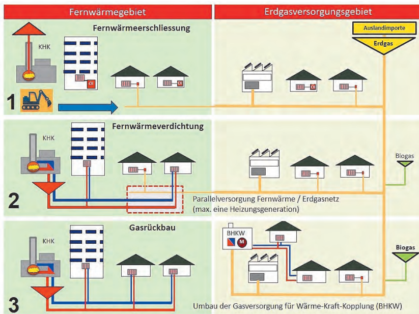
Abb. 5: Die drei Phasen der Transformation von Fernwärme- und Erdgasversorgung.
